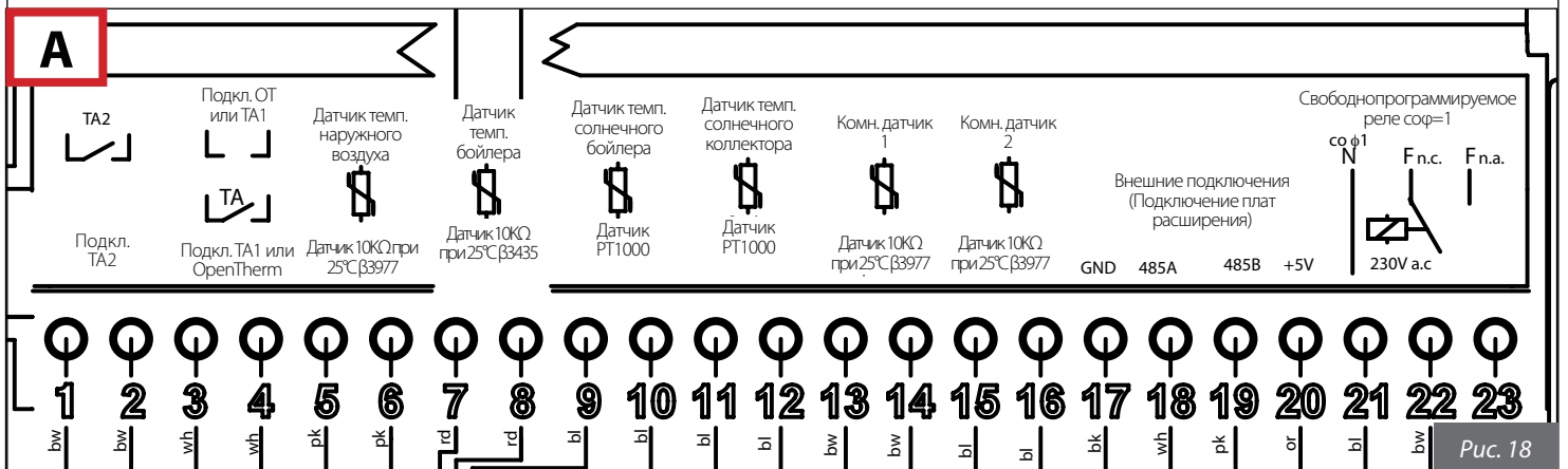
Электрическая схема подключений
